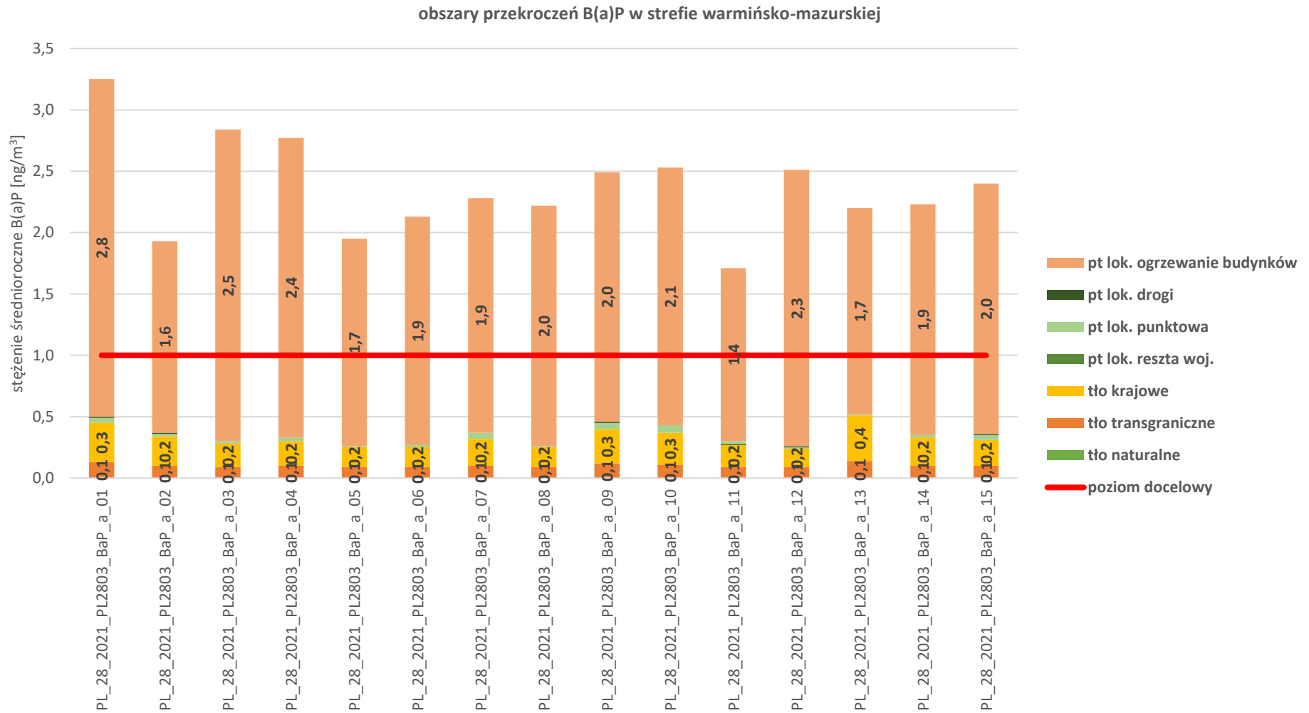
Rysunek 3. Prezentacja poziomów tła regionalnego oraz lokalnego przyrostu stężeń na terenie obszarów przekroczeń benzo(a)pirenu w strefie warmińsko-mazurskiej w 2021 roku (PL_28_2021_PL2803_BaP_a_01 do PL_28_2021_PL2803_BaP_a_15)
